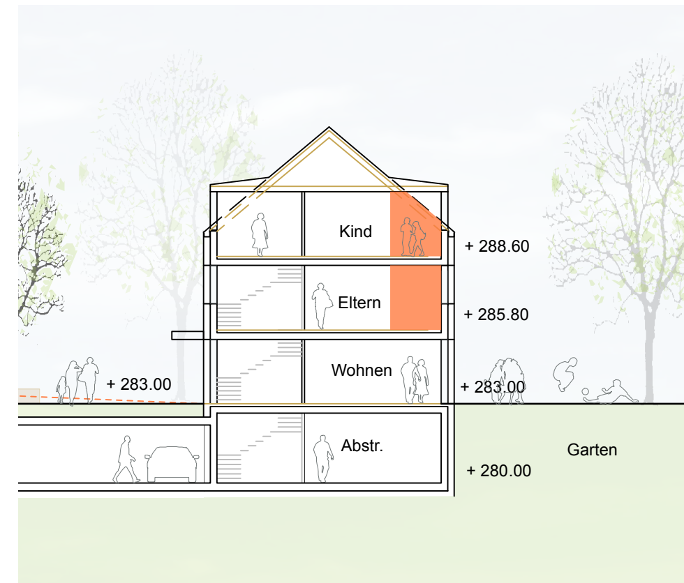
Querschnitt Variante 1
