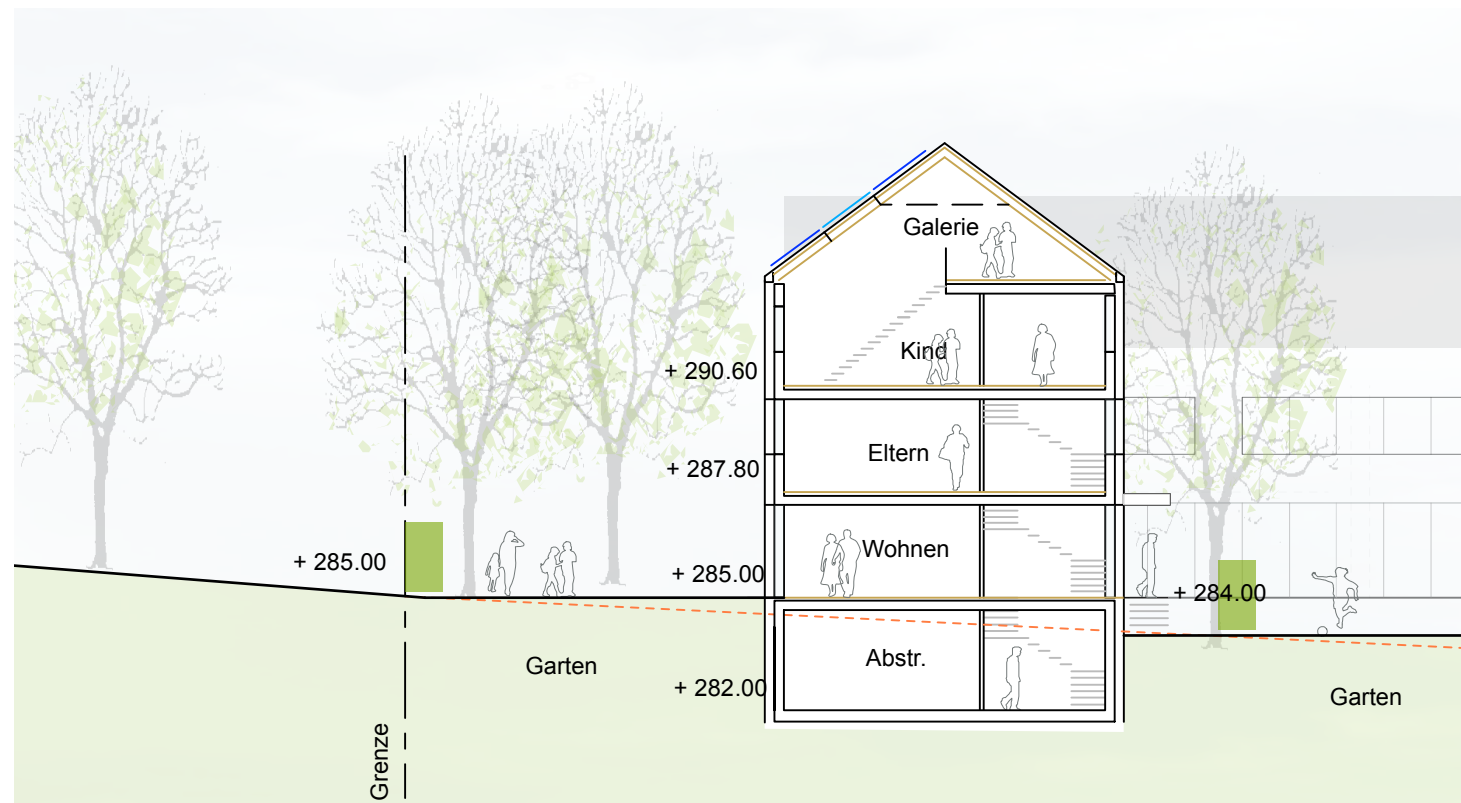
Querschnitt Variante 2
